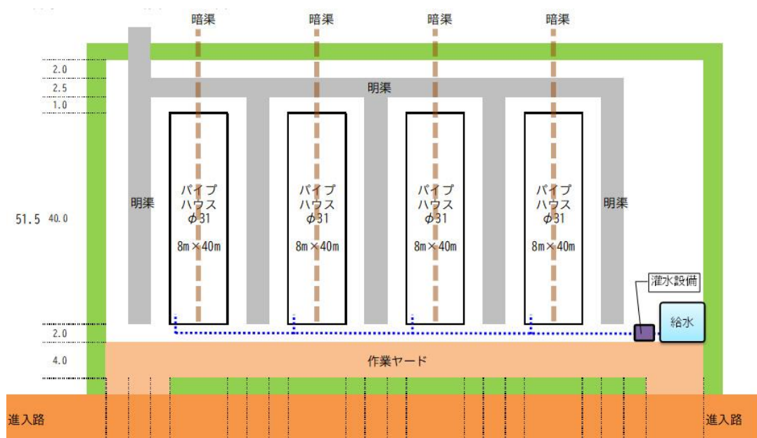
標準的なリースハウス概略図
